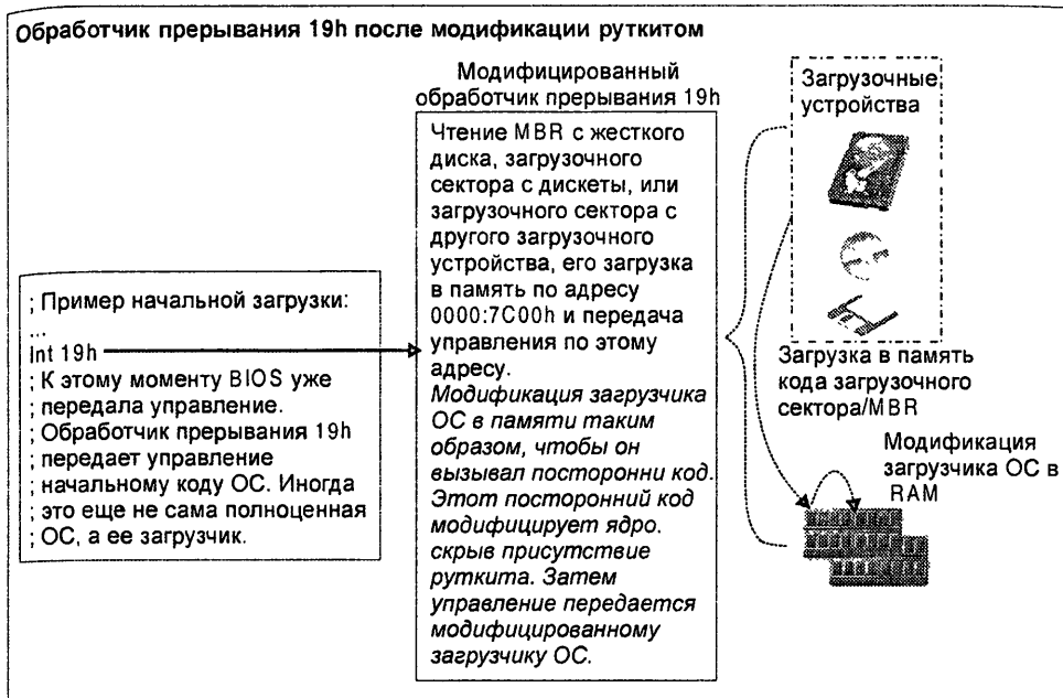
Рис. 12.9. Принцип работы модифицированного прерывания 19h
