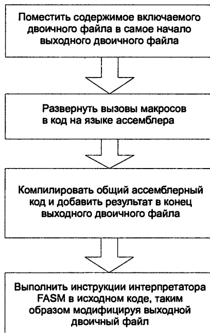
Рис. 12.13. Упрощенная схема ассемблирования BIOS PCI в FASM
