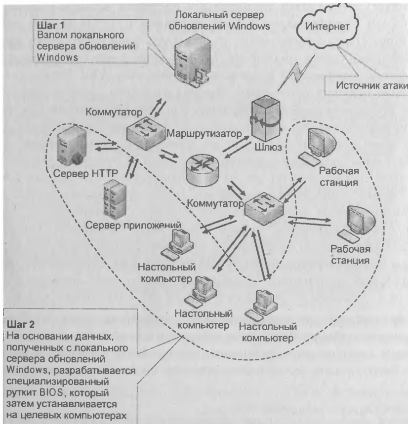
Рис. 13.2. Сценарий атаки с помощью WBEEM
