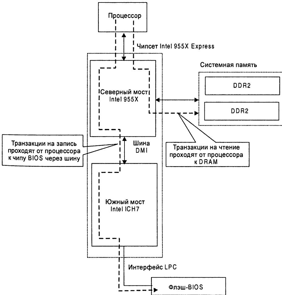
Рис. 4.5. Обращение к содержимому чипа BIOS при атрибутах доступа регистра PAM0, установленных в состоянии "только чтение"
