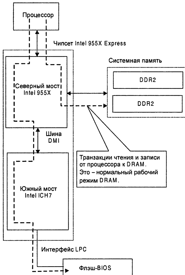
Рис. 4.6. Обращение к чипу BIOS при атрибутах доступа регистра RAM0, установленных в состоянии "штатная работа DRAM"
