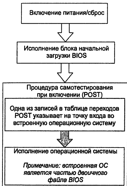
Рис. 14.1. Загрузка операционной системы, являющейся частью BIOS
