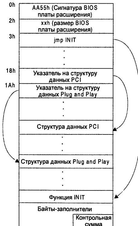
Рис. 7.3. Структура Plug-and-Play BIOS расширения PCI
