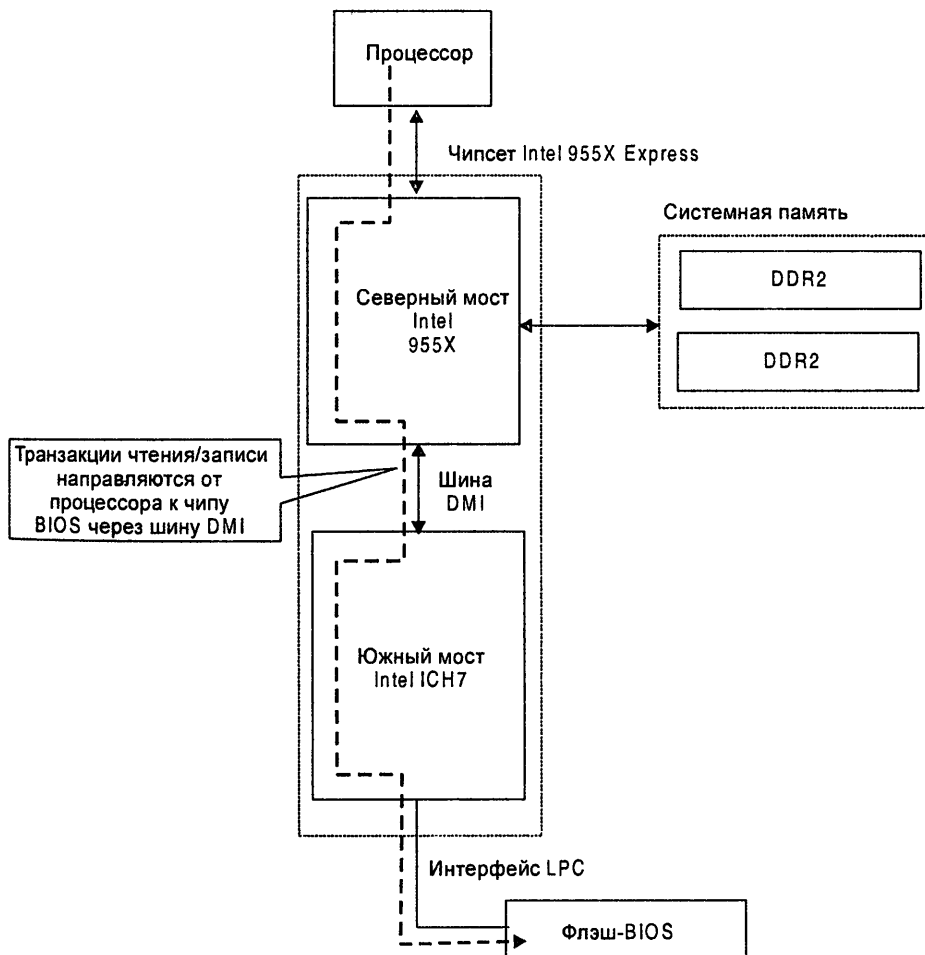
Рис. 4.3. Обращение к содержимому чипа BIOS при установке атрибутов доступа регистра PAM0 в состоянии "DRAM disabled" (DRAM заблокирована)
