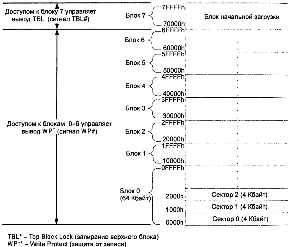
Рис. 13.1. Схема памяти чипа флэш-РОМ SST49LF004B
