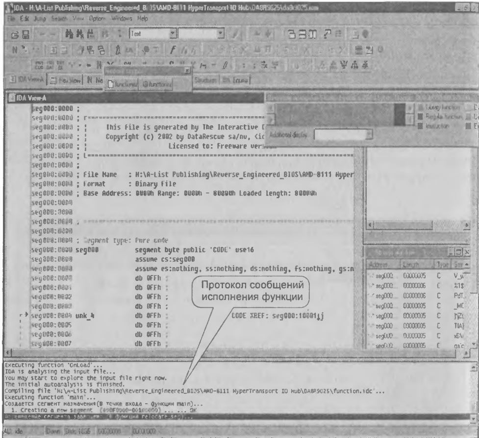
Рис. 2.10. Результат исполнения файла сценария function.idc
